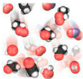
FIG. 24.3 Propagação radical
