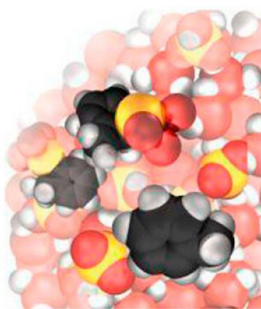
FIG. 16.4 Enxofre ligando-se
