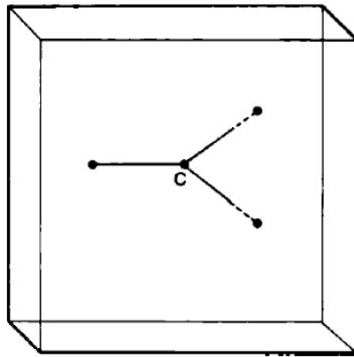
Figura 5a. Em C, a junção de ondas de Schrödinger contrai-se, caracterizando a esquizofrenia, e o seu vetor no espaço de configuração divide-se, uma vez que se prevê que a partícula execute dois resultados mutuamente exclusivos.
