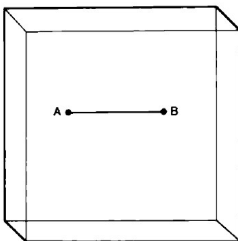
Figura 4. A representa o estado inicial da partícula; B representa o seu estado ao longo do tempo (descrito pela equação de Schrödinger).
